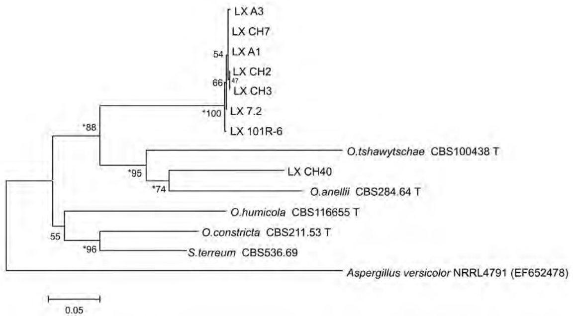
Figure 5. Relations phylogénétiques entre les isolats d' Ochoconis spp. provenant de Lascaux et les isolats de référence (CBS). Analyse basée sur l'alignement multiple de la région ITS, réalisé en comparant 680 nucléotides. L'arbre a été établi par la méthode de neighbour-joining utilisant 1.000 répliques. Les astérisques indiquent nœuds de l'arbre, obtenus en utilisant l'algorithme d'Evolution Minimale et Parcimonie Maximale UPGMA. La barre représente 0.05 changement de nucléotides par position.
